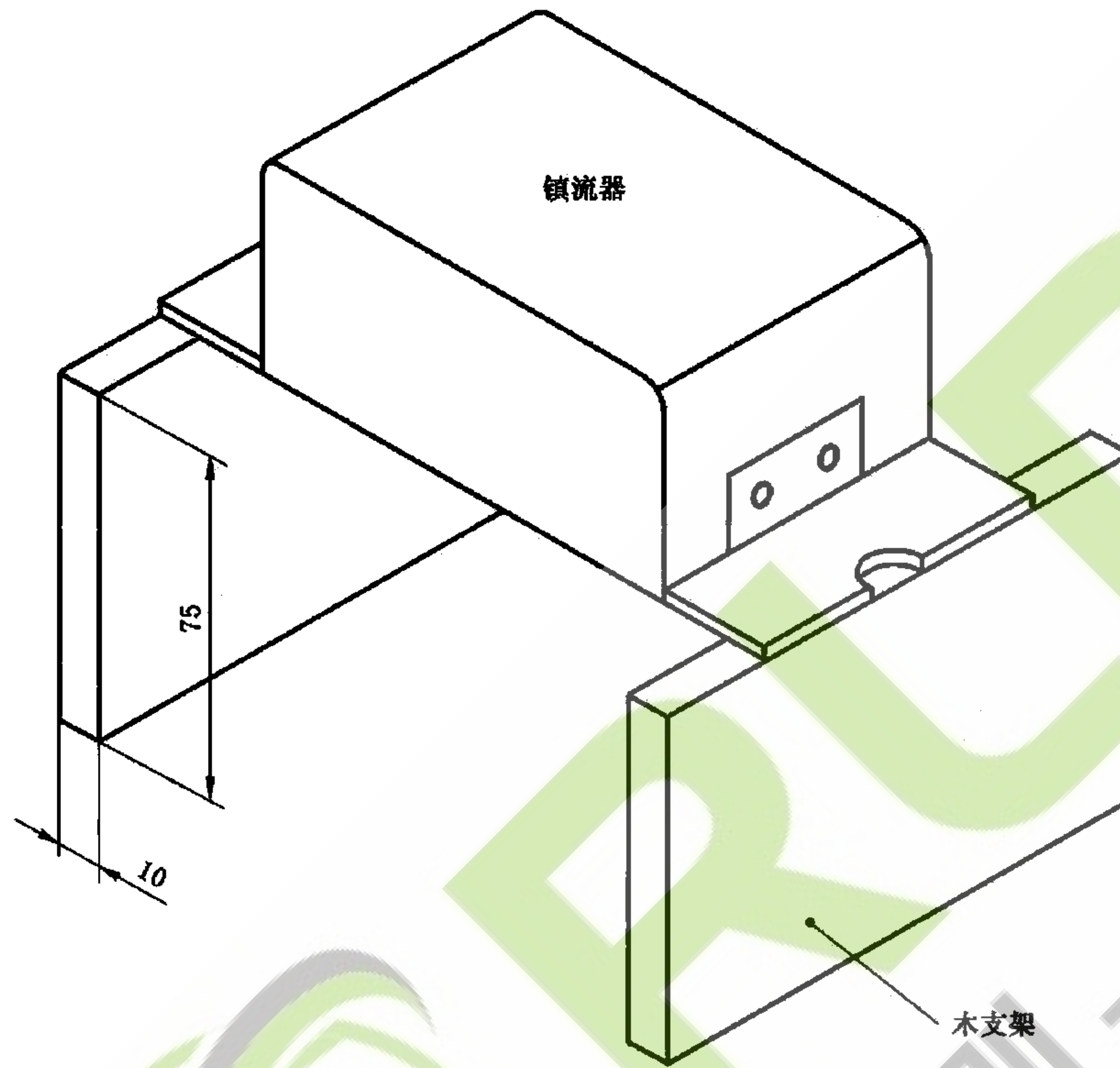
图 H.1 加热试验样品配置图
